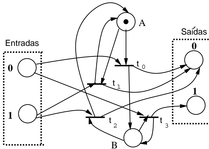
Figura 2.12: Detector de Seqüência
