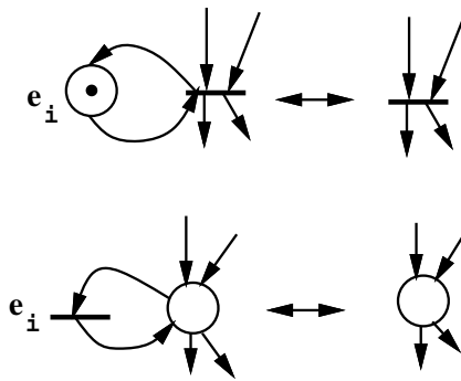
Figura 3.32: Reduções - Eliminação de Self-loop
