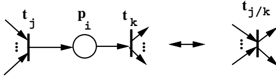
Figura 3.29: Reduções - Fusão de Transições Série
