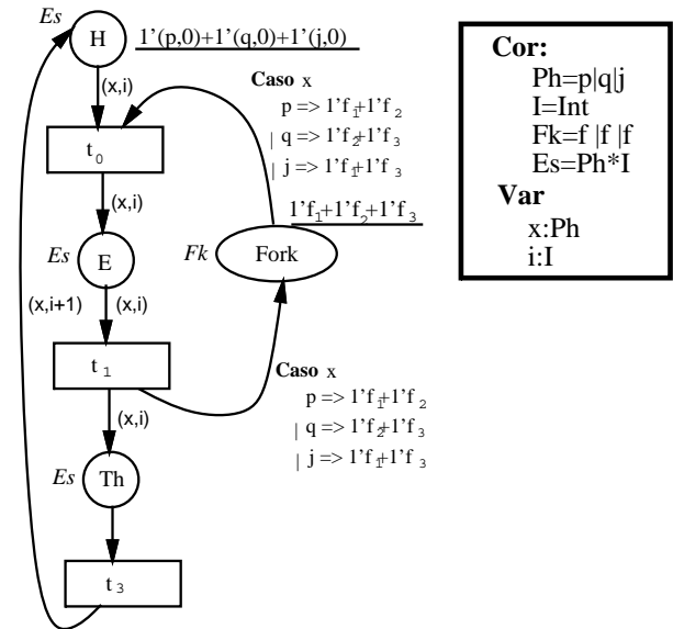
Figura 4.7: Jantar dos Filósofos - Modelo com Redes Coloridas
