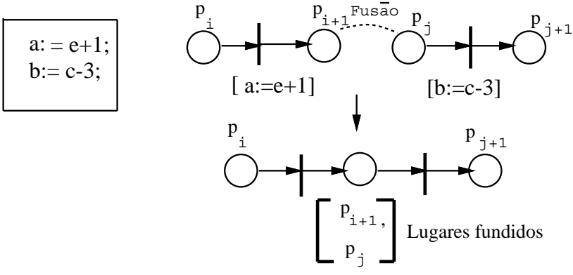
Figura 2.23: Fusão dos Lugares
