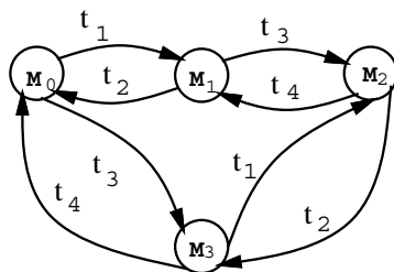
Figura 1.13: Grafo das Marcações Acessíveis
