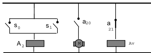
Figura 5.20: Diagrama Elétrico
