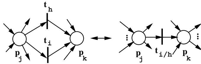
Figura 3.31: Reduções - Fusão de Transições Paralelas
