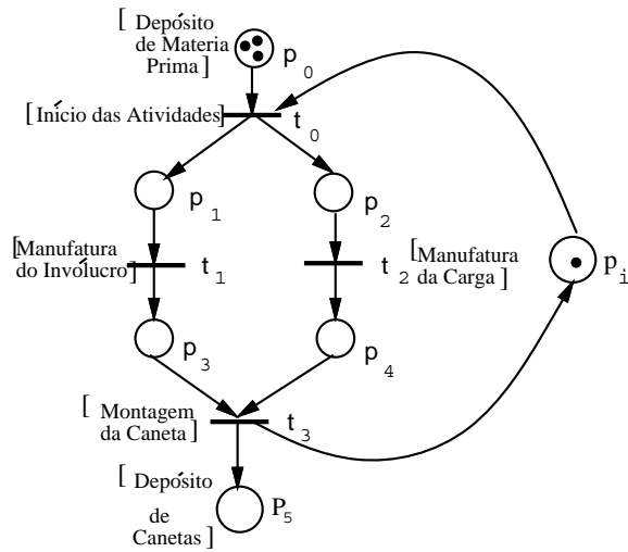
Figura 2.8: Atividades Paralelas
