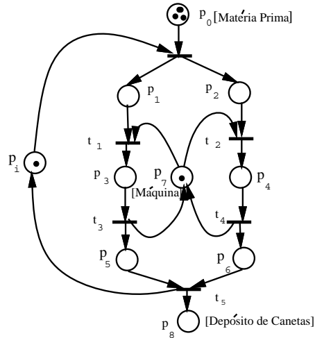
Figura 2.9: Exclusão Mútua
