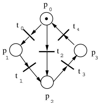
Figura 3.1: Rede N
