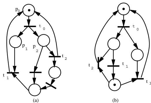
Figura 3.16: Repetitividade
