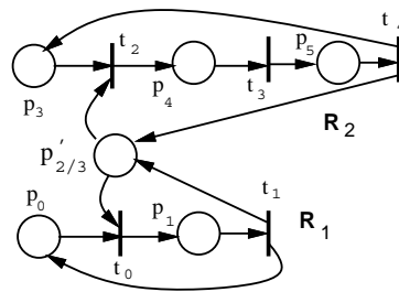
Figura 3.27: Rede R
