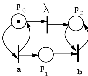
Figura 1.17: Rede Rotulada
