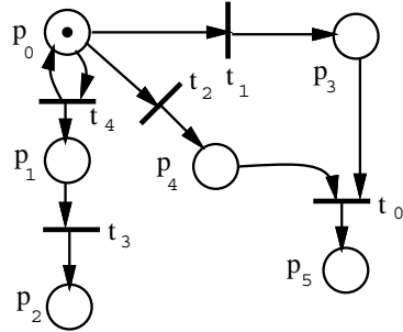
Figura 3.8: Níveis de Liveness
