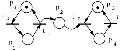
Figura 3.15: Rede não Conservativa
