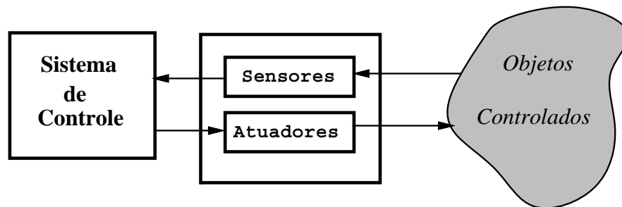
Figura 5.18: Sistema de Controle Seqüencial
