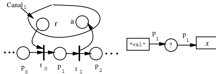
Figura 5.2: Input
