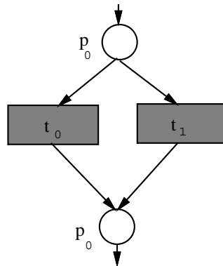
Figura 4.8: Superpágina
