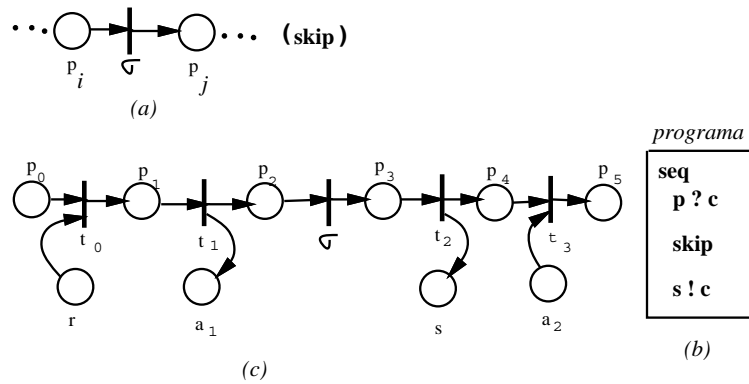
Figura 5.4: Skip
